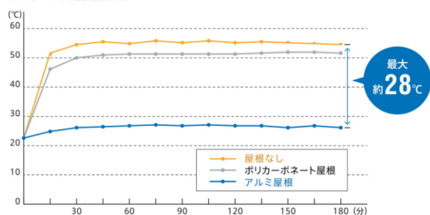
人工木デッキ表面温度比較
